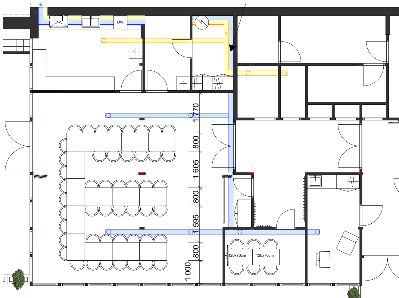
1:100 1. Etasje
